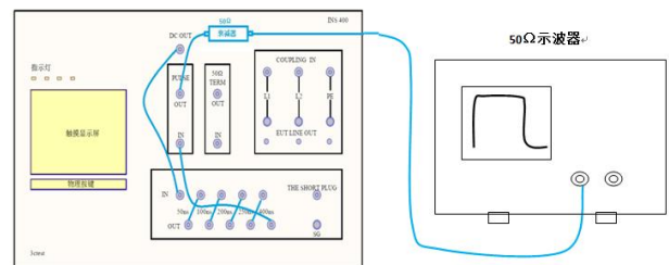
2、典型测试连接示意图 (差模 L1-L2):
