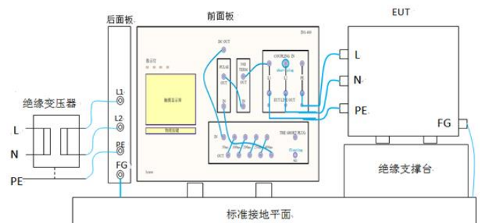
2、典型测试连接示意图 (差模 L1-L2):
