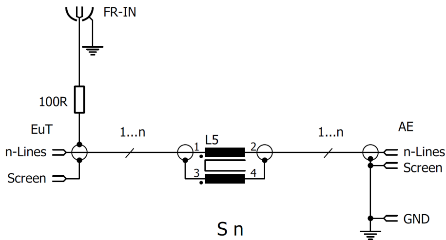
Bild 4: Prinzipschaltbild CDN S4 XLR4 Fig. 4: principal circuitry CDN S4 XLR4
