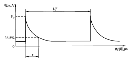
干扰电压 A 波和 C 波
