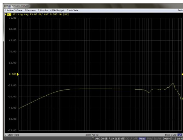
TWCM-500 宽带电流监测钳 s21 曲线*
